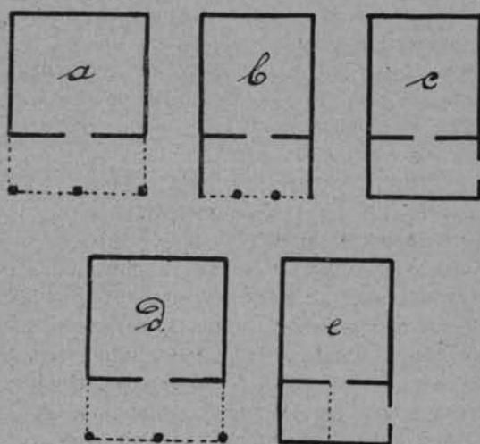
PLANY CHAT JEDNOIZBOWYCH PLECIONYCH I CIOSANYCH.
