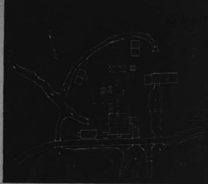
Orientacyjny szkic walcowni w Koniecpolu, 1 — szopa walcownicza, 2 — gwoździarnia, 3, 4 — warsztat, odlewnia i kotłarnia, 5 — piec do topienia miedzi, 6 — piece grzejne, 7 — skład gotowych blach, 8 — pomieszczenie gospodarcze, 9 — kanał, 10 — koło wodne, 11 — trak, 12 — domy robotnicze.
