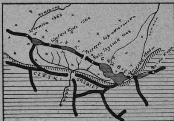
Geologiczny szkic Karkonoszy.
